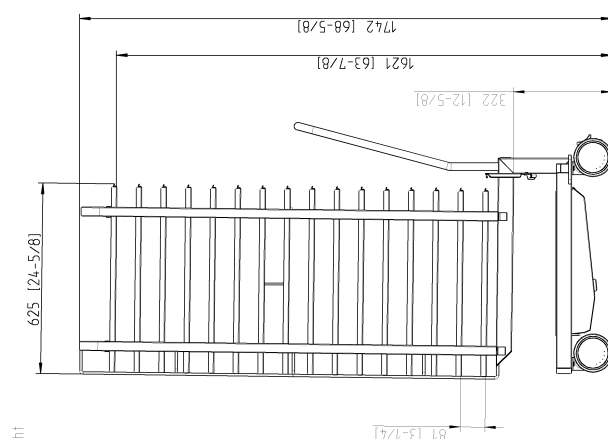
Seitenansicht side view
