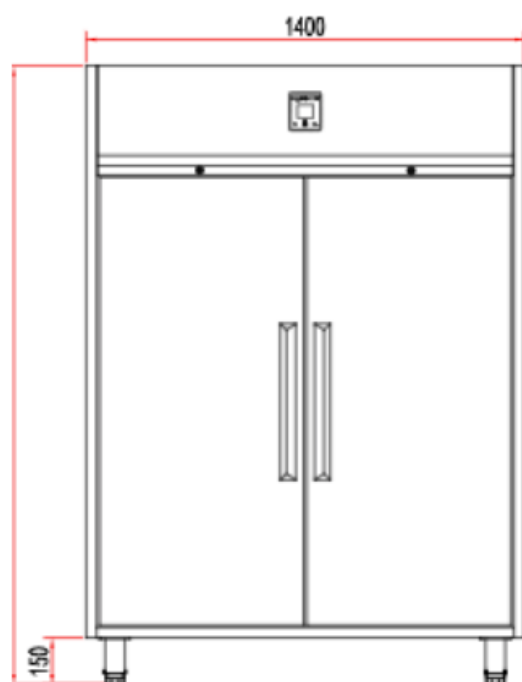
ELEVATION 前视图
